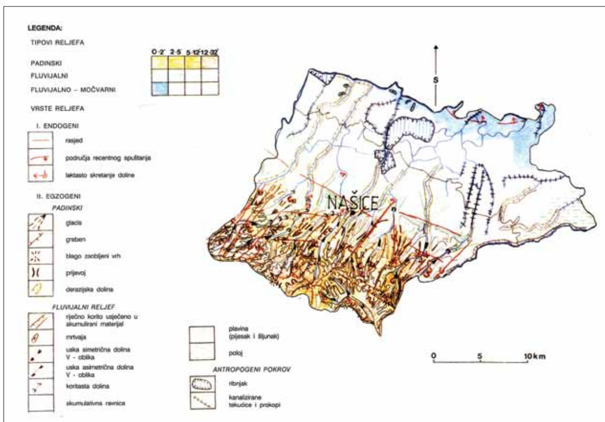
Sl. 7 Geomorfološka karta (prema Kovač 2001).
