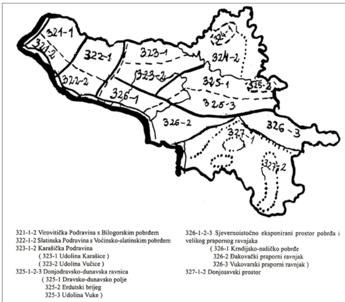
Sl. 4 Našički kraj prema Nasctu uvjetno homogene regionalizacije istočnohrvatske ravnice (prema Kovač 2001: 14, sl. 4).
