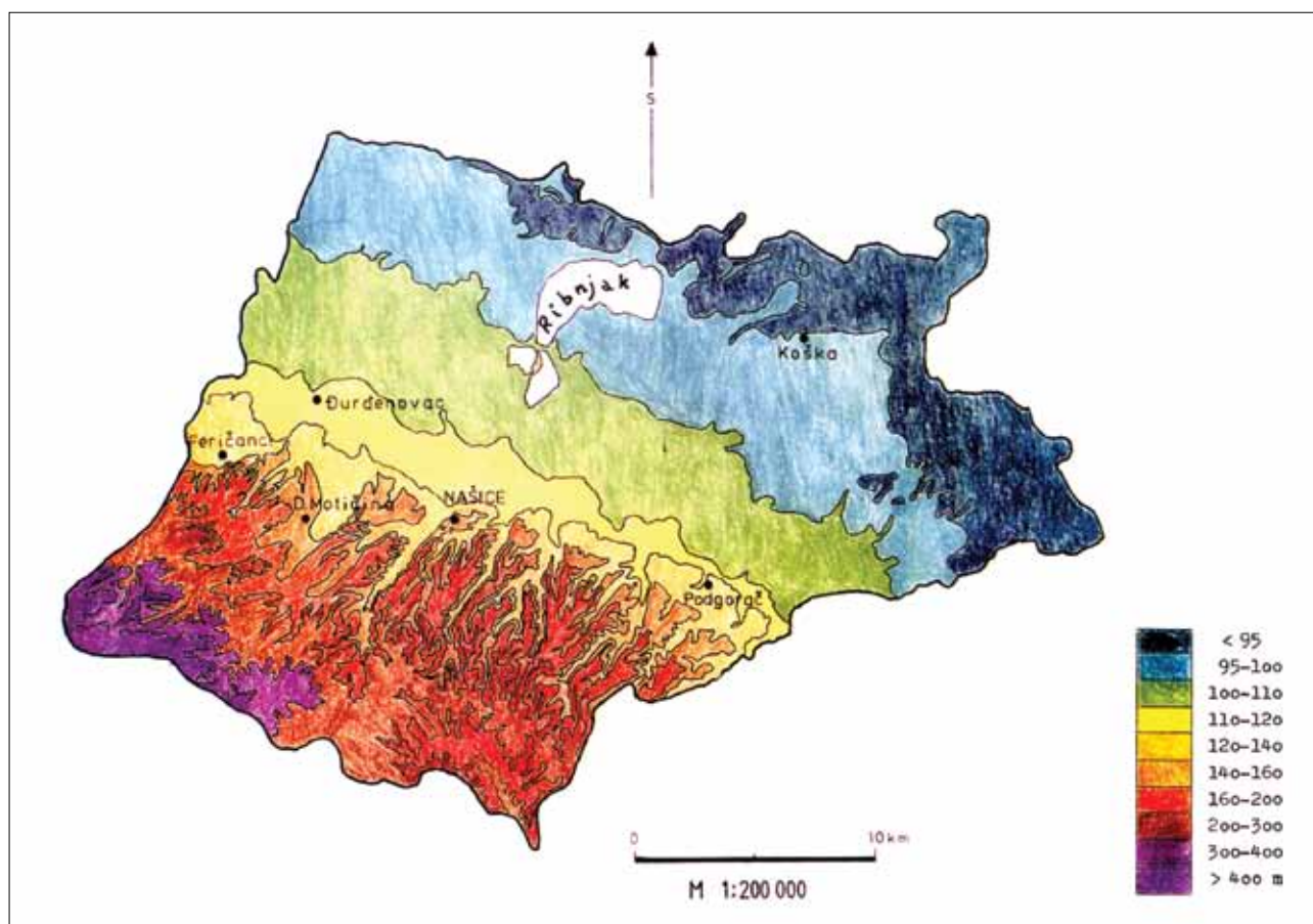
Sl. 8 Hipsometrijska karta (prema Kovač 2001).
