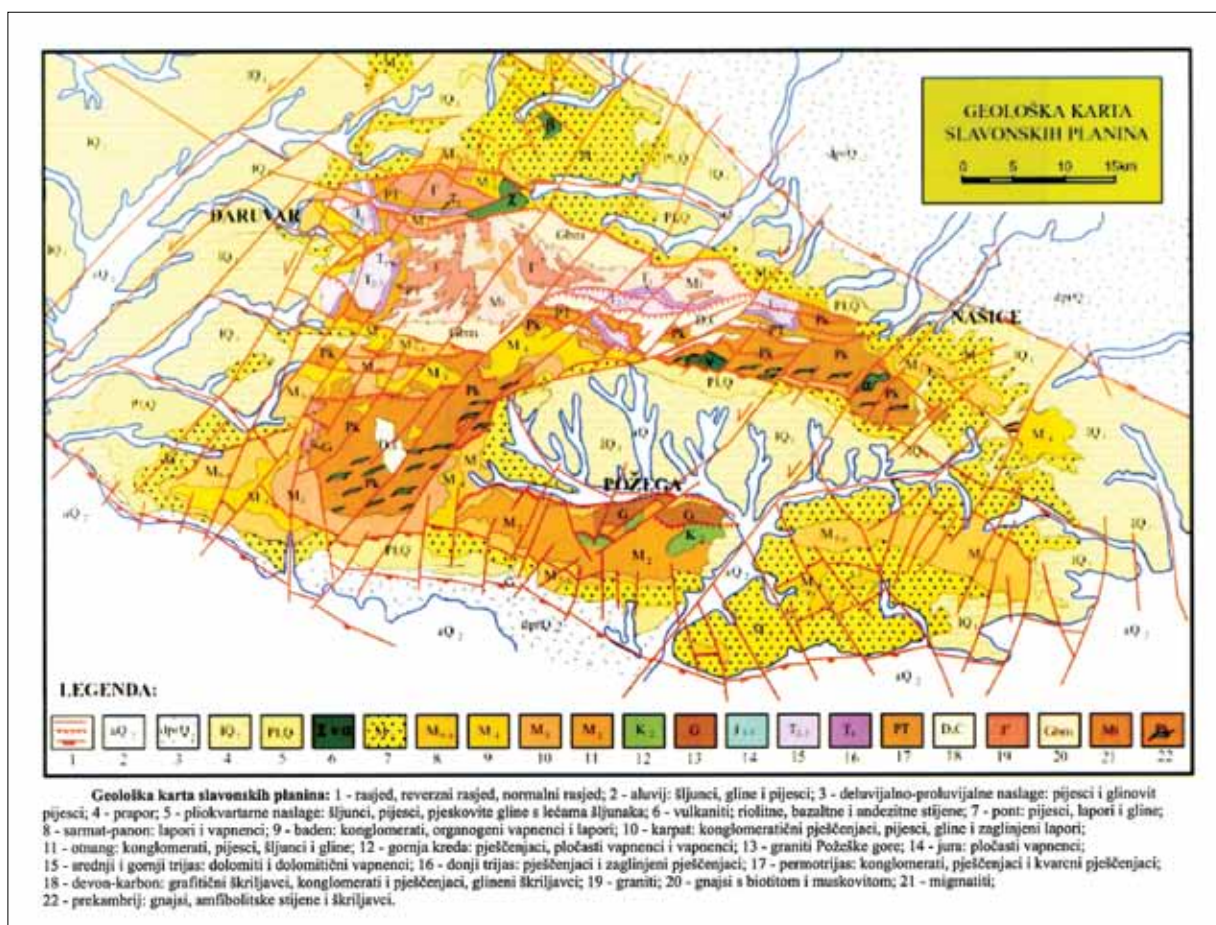
Sl. 6 Geološka karta slavonskih planina (Jamičić 2001: sl. 1).
