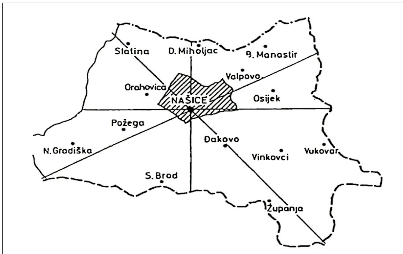
Sl. 2 Našički kraj, središnji položaj u istočnoj Hrvatskoj (prema Kovač 2001: 13, sl. 2).
