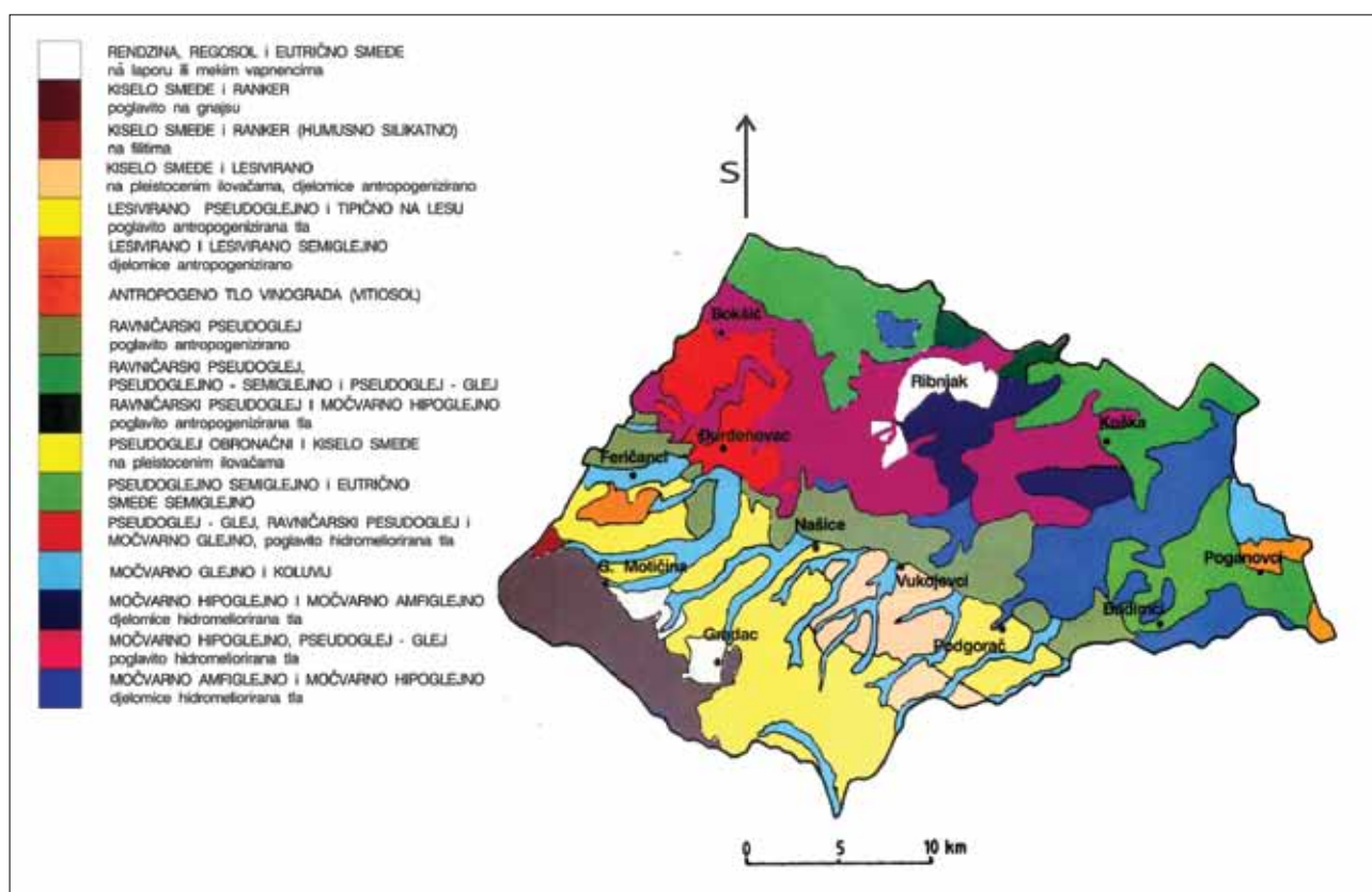
Sl. 9 Pedološka karta našičkog područja (prema Kovač 2001).
