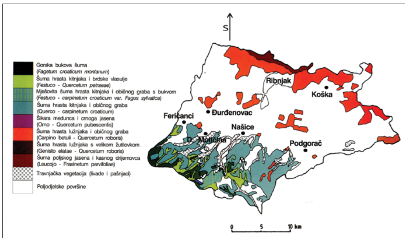
Sl. 10 Vegetacijska karta našičkog područja (prema Kovač 2001).
